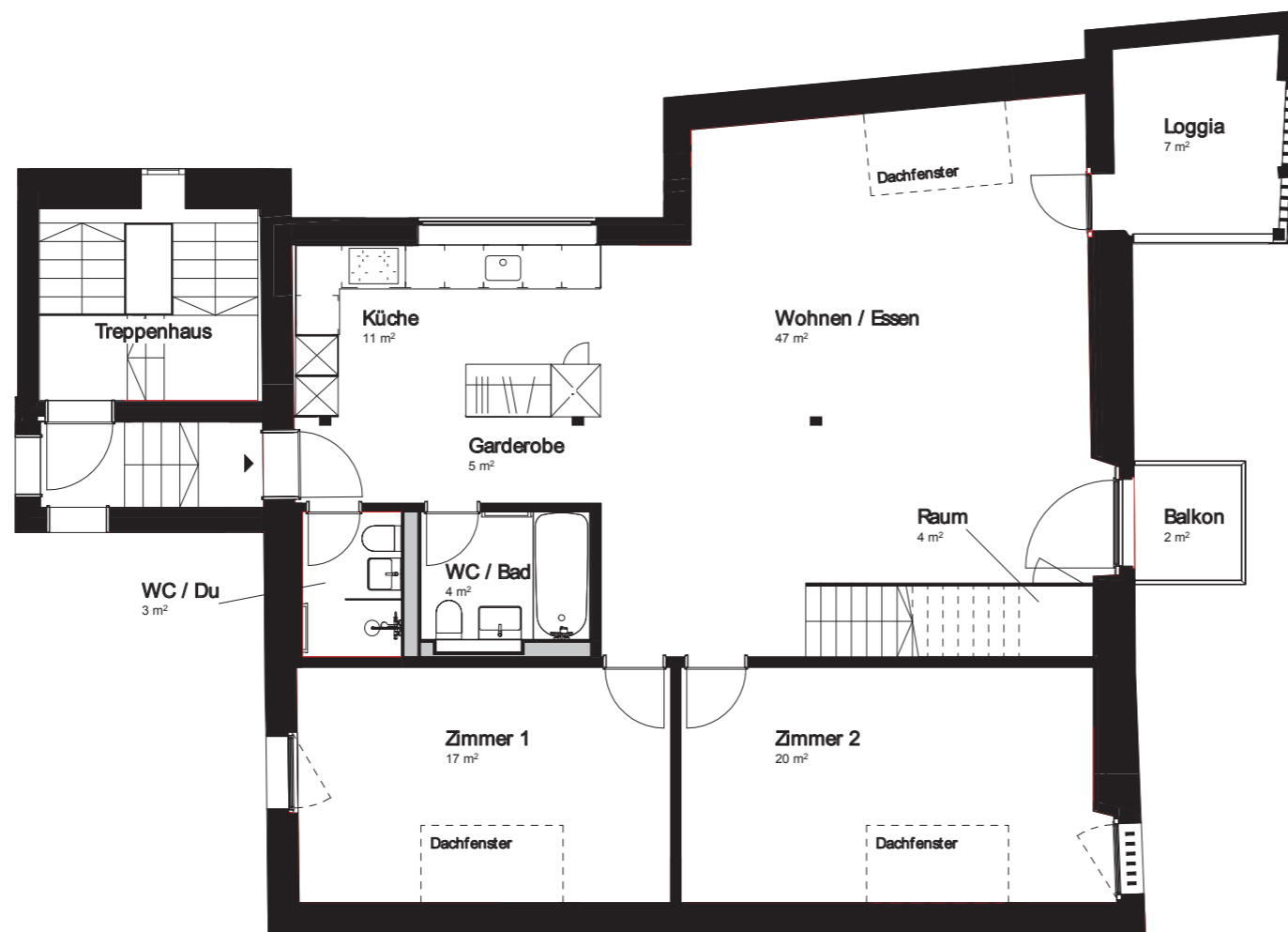
DACHGESCHOSS
